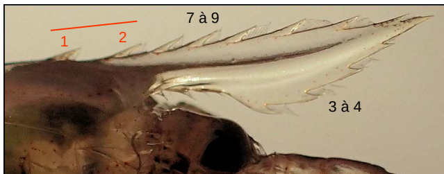
Palaemon longirostris
