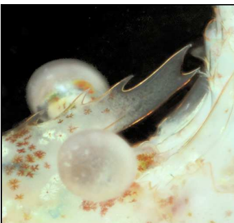
Eualus occultus
